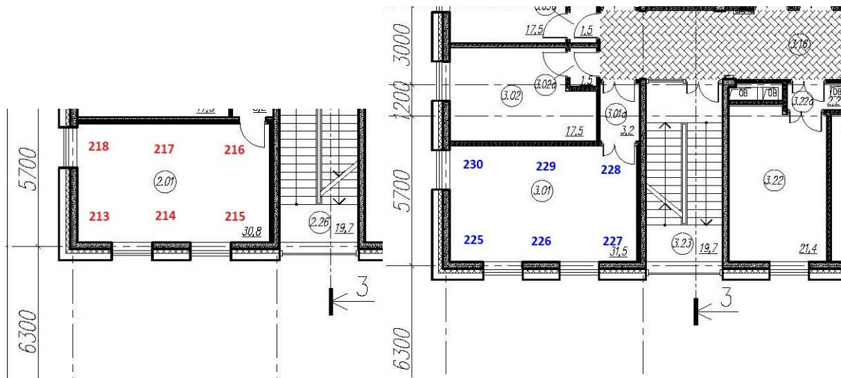
Рисунок 2.1 – Эскиз исследуемой ограждающей конструкции с нанесением источников шума и указанием мест установки и ориентации микрофонов, порядковые номера точек измерения
