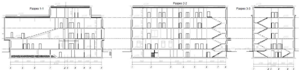
Рисунок 1.1 – Место проведения измерений. Детская школа искусств (Разрез)
