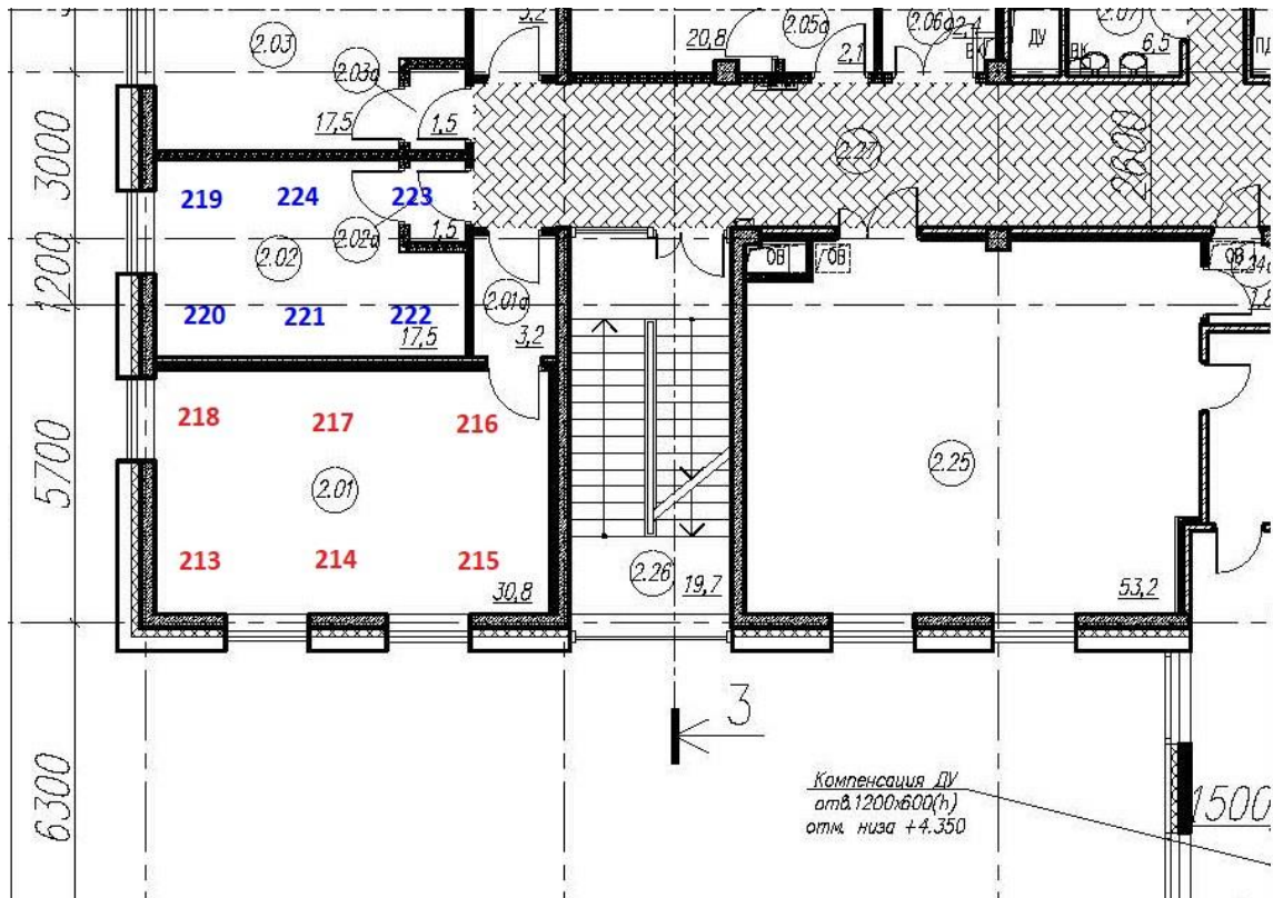
Рисунок 2.1 – Эскиз исследуемой ограждающей конструкции с нанесением источников шума и указанием мест установки и ориентации микрофонов, порядковые номера точек измерения
